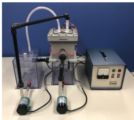
UH-1 型生成装置
