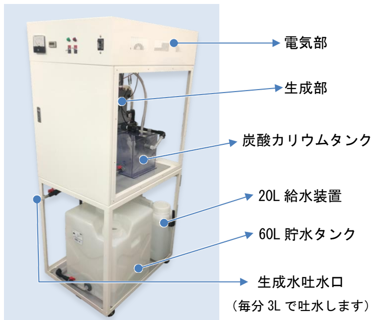
SARES II-300-N 型
